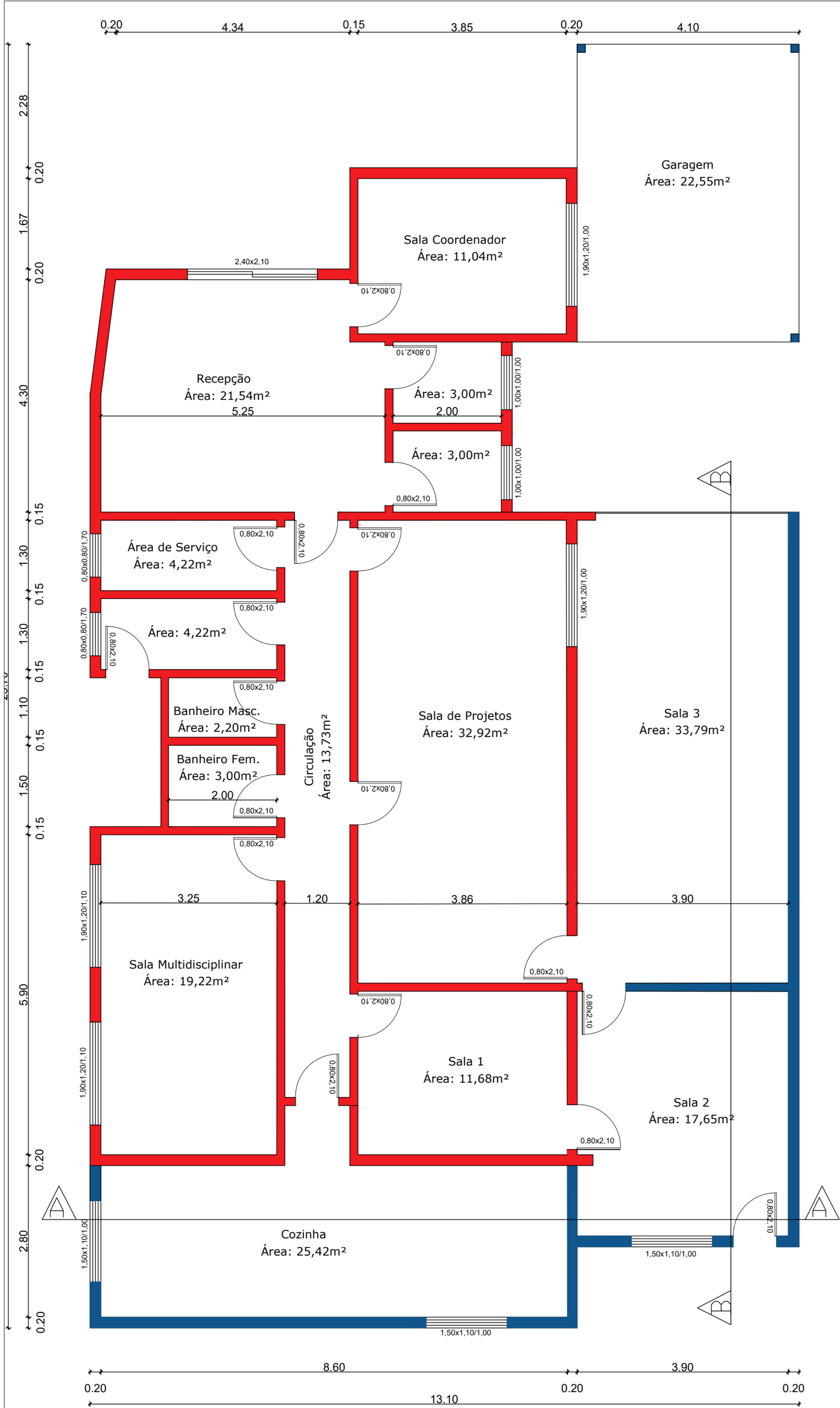
PLANTA BAIXA ESC. 1/50
