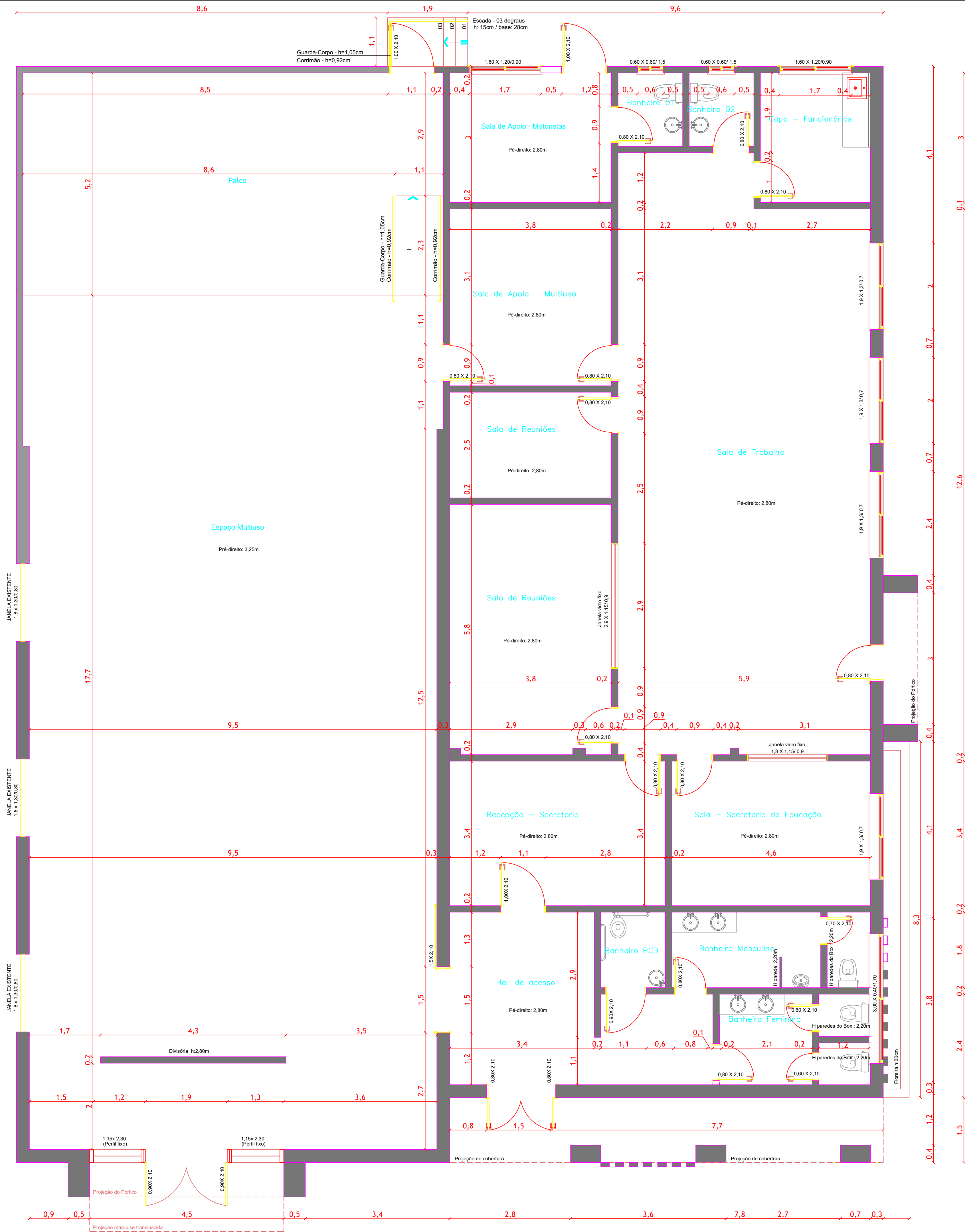
PLANTA BAIXA TÉCNICA ESCALA: 1:50
