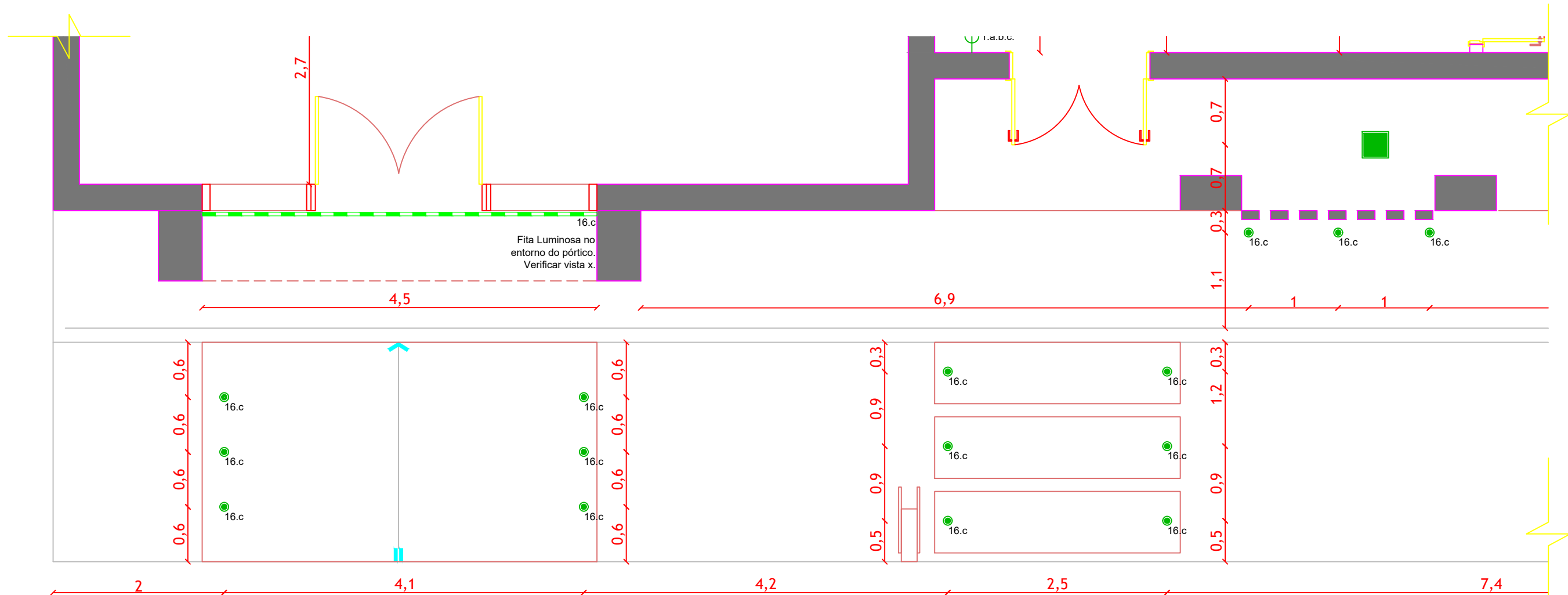
PLANTA BAIXA LUMINOTÉCNICA - ÁREA EXTERNA ESCALA: 1:50
